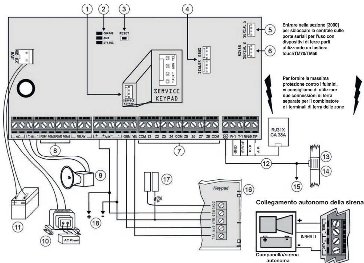
Figura 3: collegamento cavi alla centrale EVOHD+.
