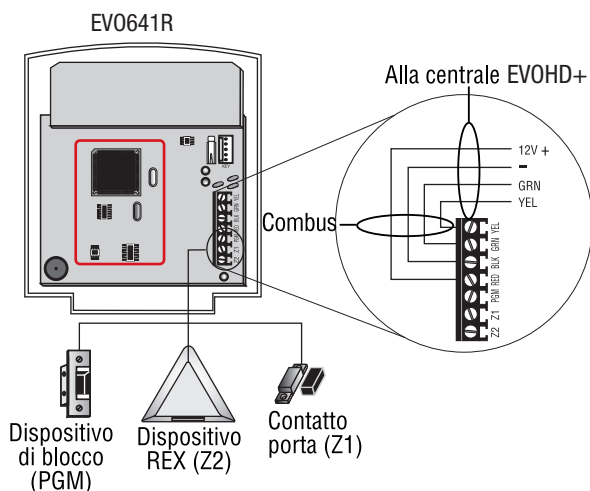
Figura 24: Collegamenti Controllo Accesso
