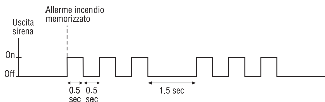
Figura 14: Uscita di Sirena durante l'Allarme Incendio
