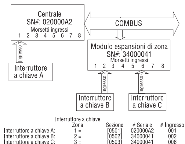
Figura 15: esempio numerazione di inseritore a chiave
