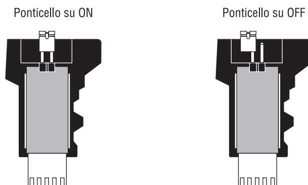
Figura 21: PMC-4 Configurazione di Ponticello
